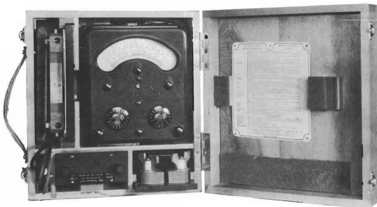
A.P.48A AVOMETER 48A
